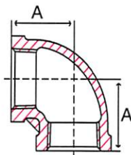
Fig. S3014E & S3016E - 90° Elbow
